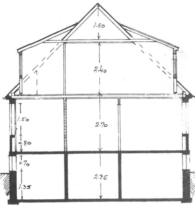
DVERSK. A-A
